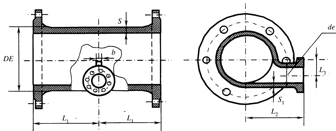
Рисунок Б.23 — Выпуск фланцевый
