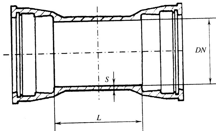
Рисунок Б.20 — Двойной раструб
