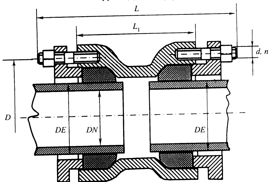
Рисунок Б.21 — Двойной раструб компенсационный
